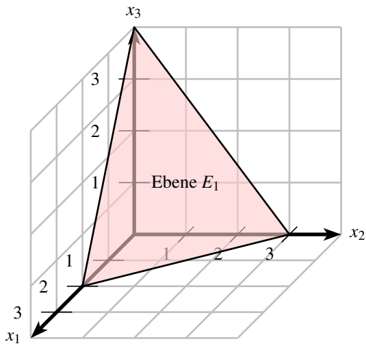
Abb. 1: E_1 : 6x_1 + 4x_2 + 3x_3 = 12
